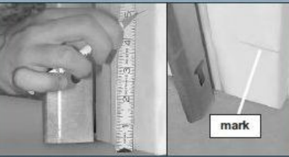
FIG 4-1 Mark door frame.
